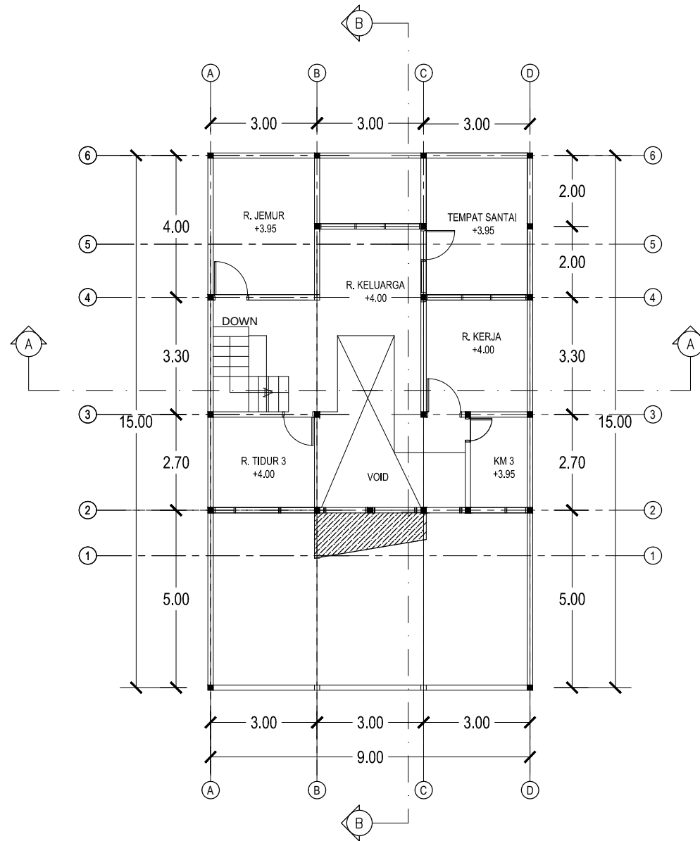
DENAH RENCANA LT. 2
