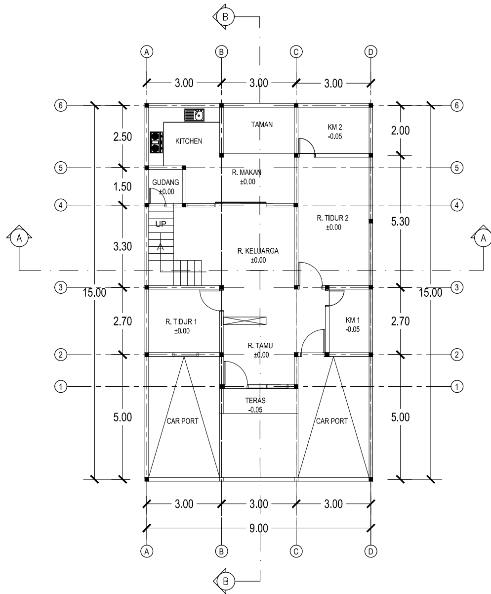
DENAH RENCANA LT. 1
